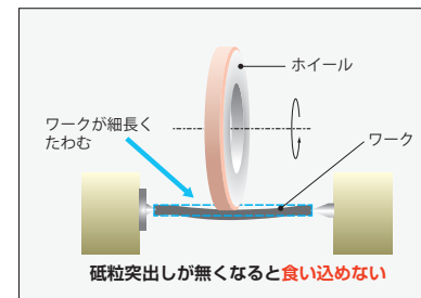
図2 超硬の円筒研削での問題点
