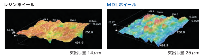
図10 試験結果
