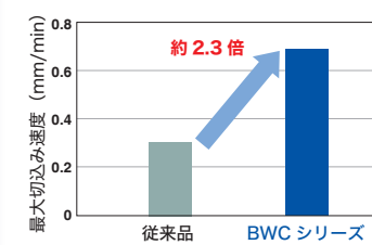
図4 試験結果
