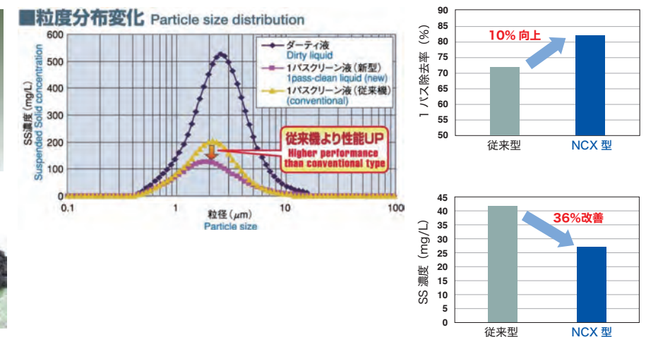
図13 試験結果
