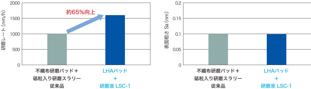
図9 試験結果
