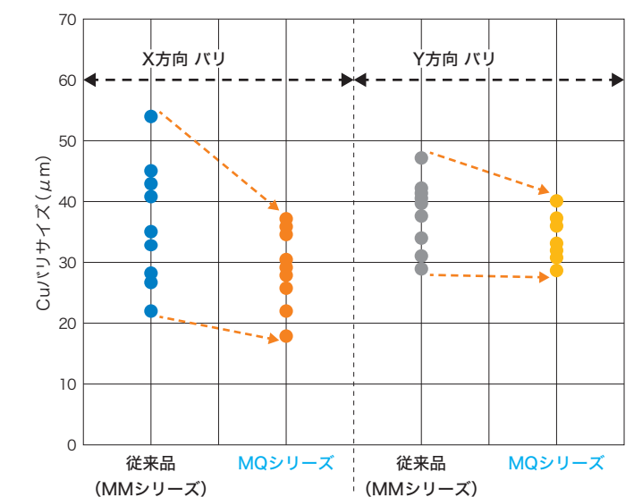
図16 試験結果
