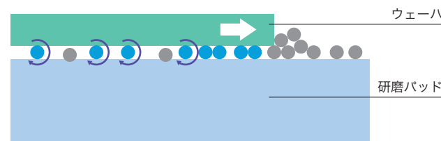
図12 LHAパッドの砥粒の作用
