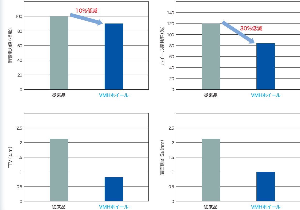
図5 試験結果
