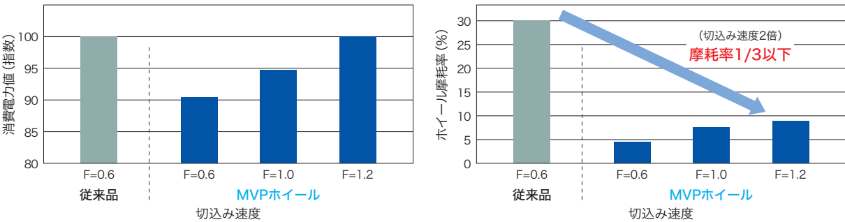
図3 試験結果
