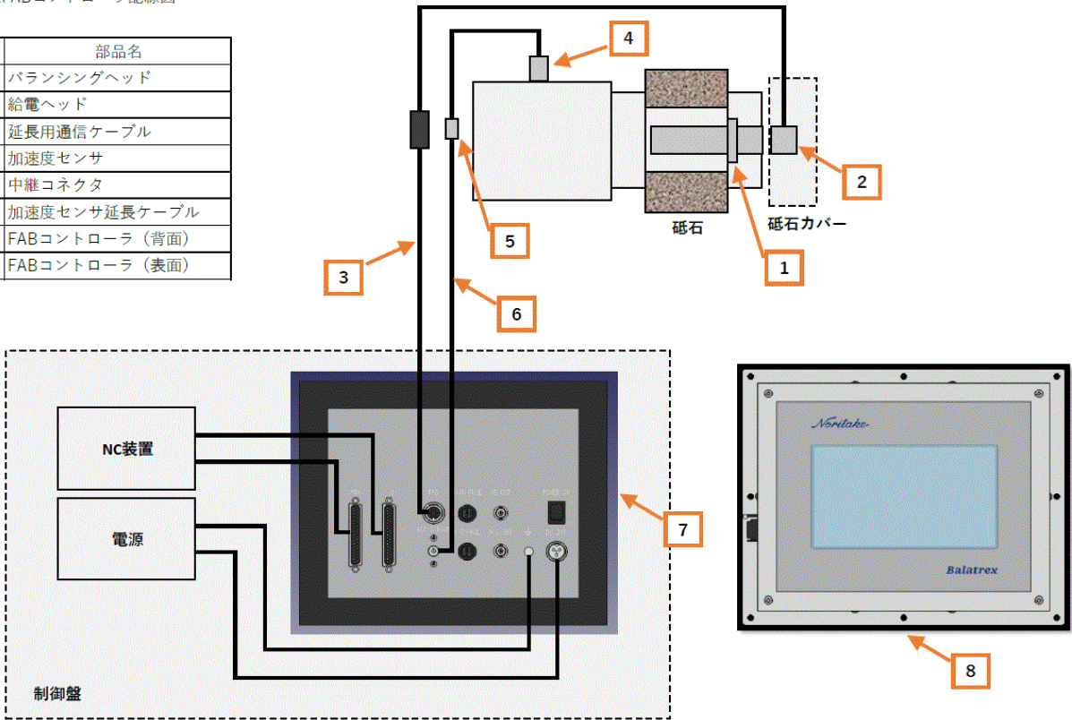
φ42FABコントローラ配線図
