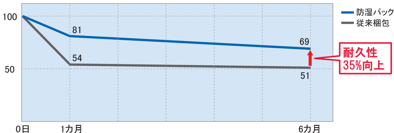
防湿パックと従来梱包砥石の耐久性(指数表示)※スーパーリトル1.0の実験データ
