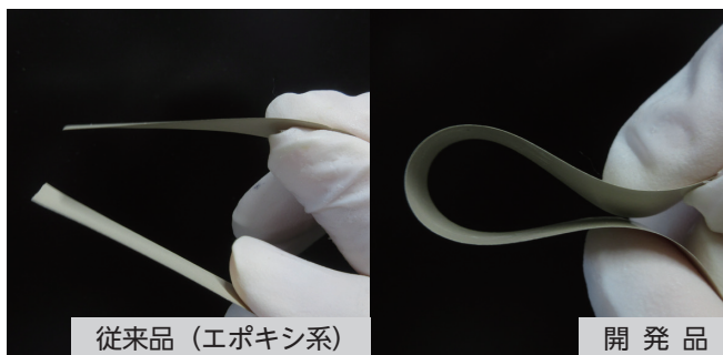
▲従来品との柔軟性比較（試験：200℃以上で10時間焼成）
